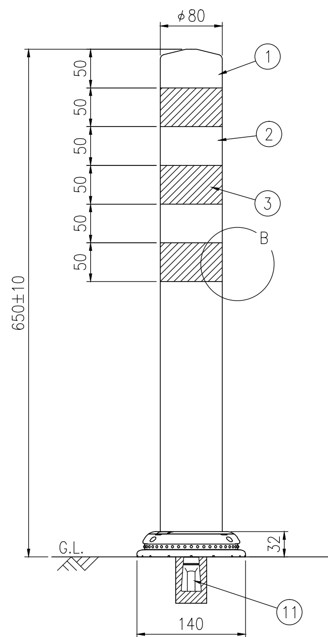
設置図 S=1/5
