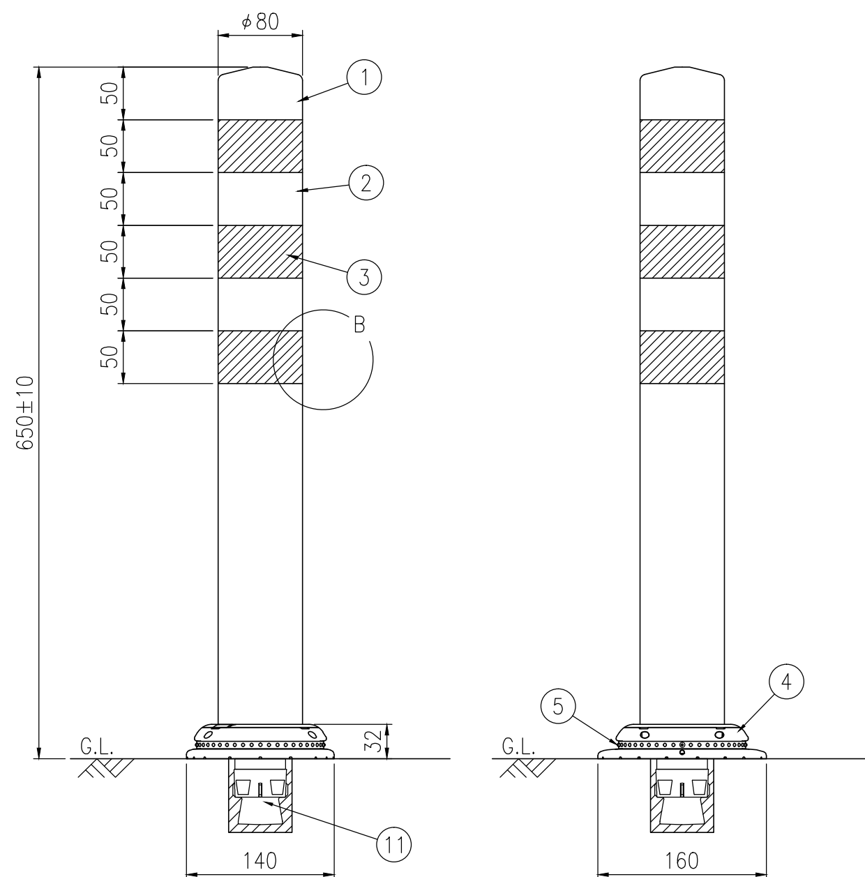
設置図 S=1/5
