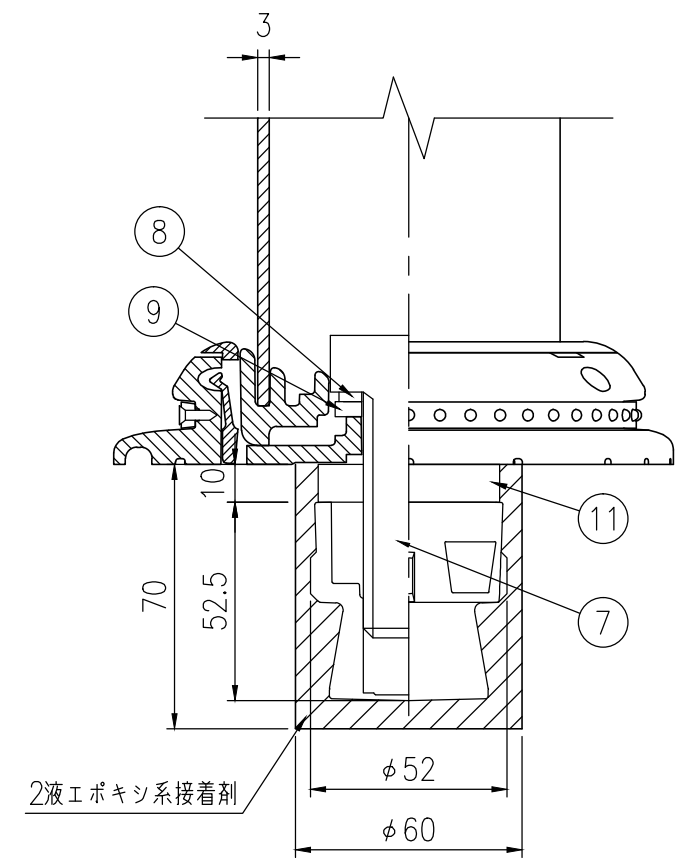
A-A半断面図 S=1/2
