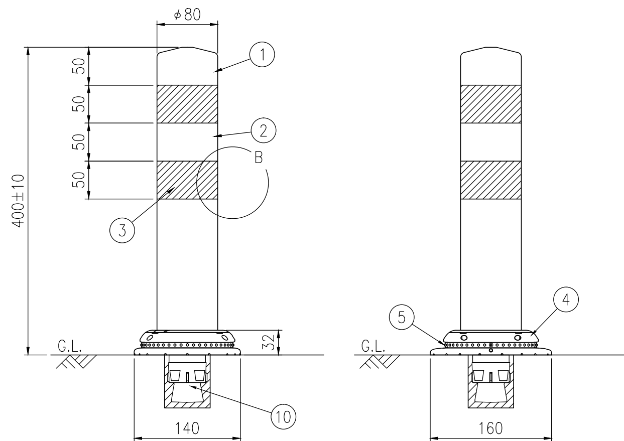
設置図 S=1/5
