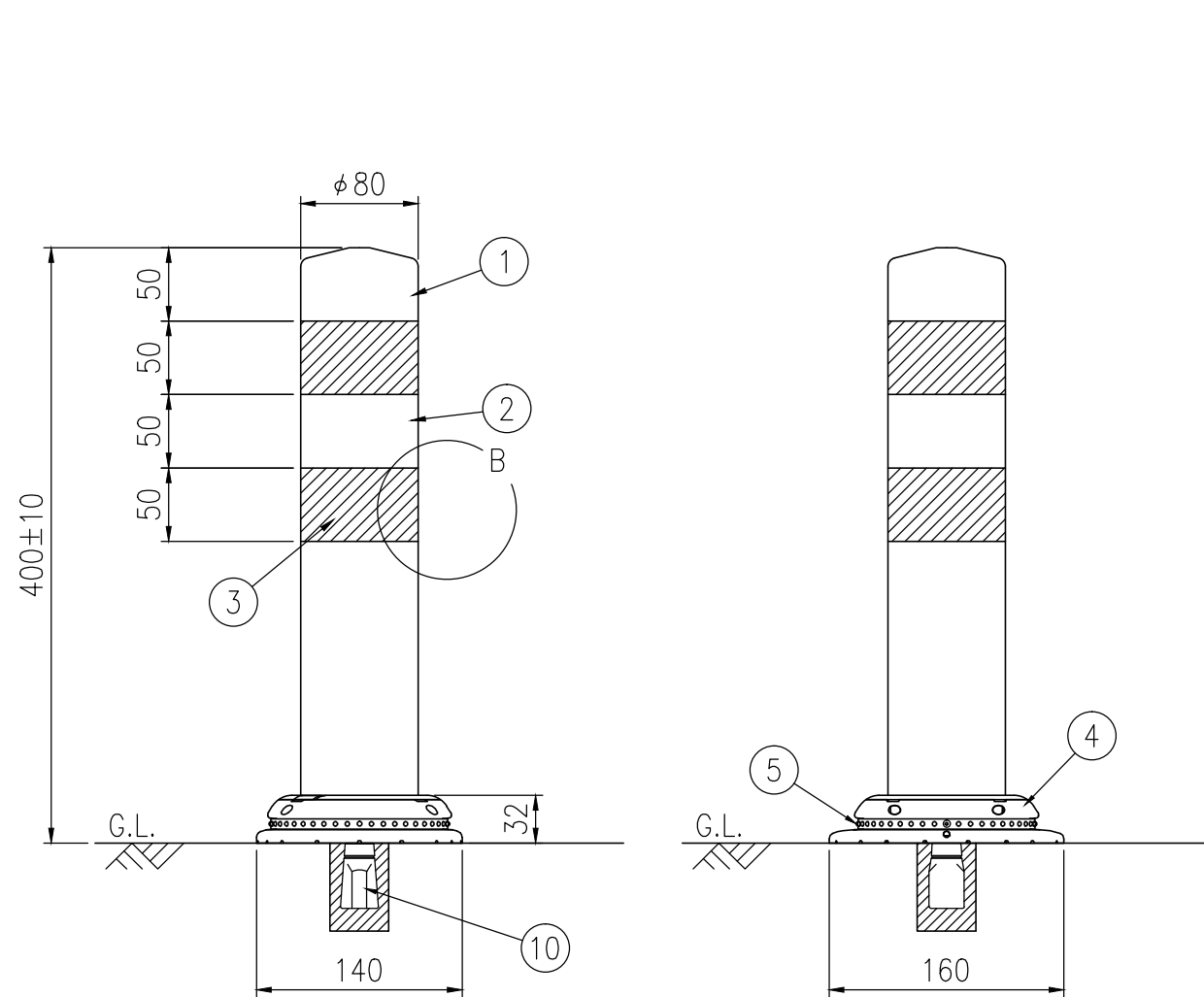
設置図 S=1/5
