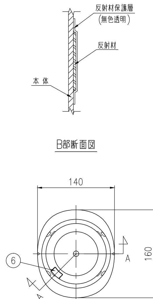
平面図 S=1/4
