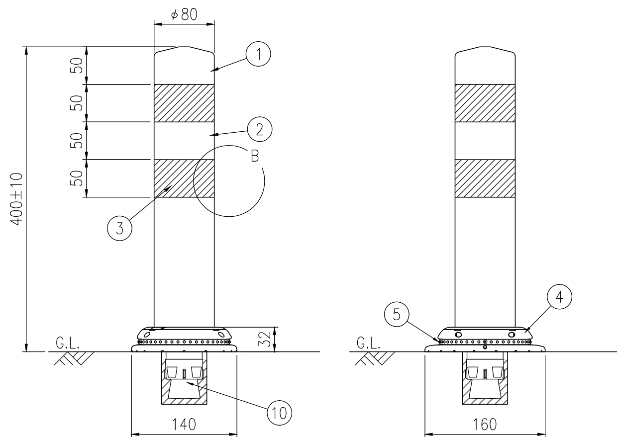
設置図 S=1/5
