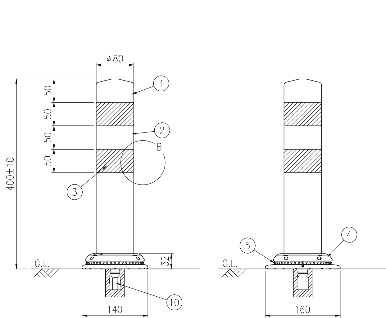
設置図 S=1/5
