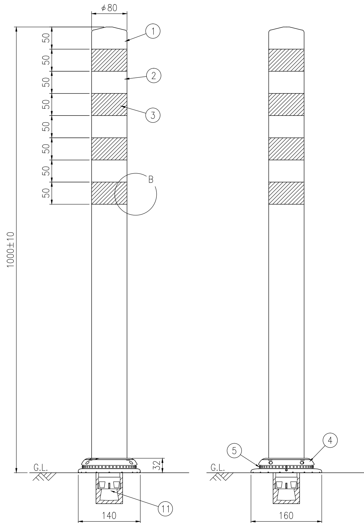
設置図 S=1/5
