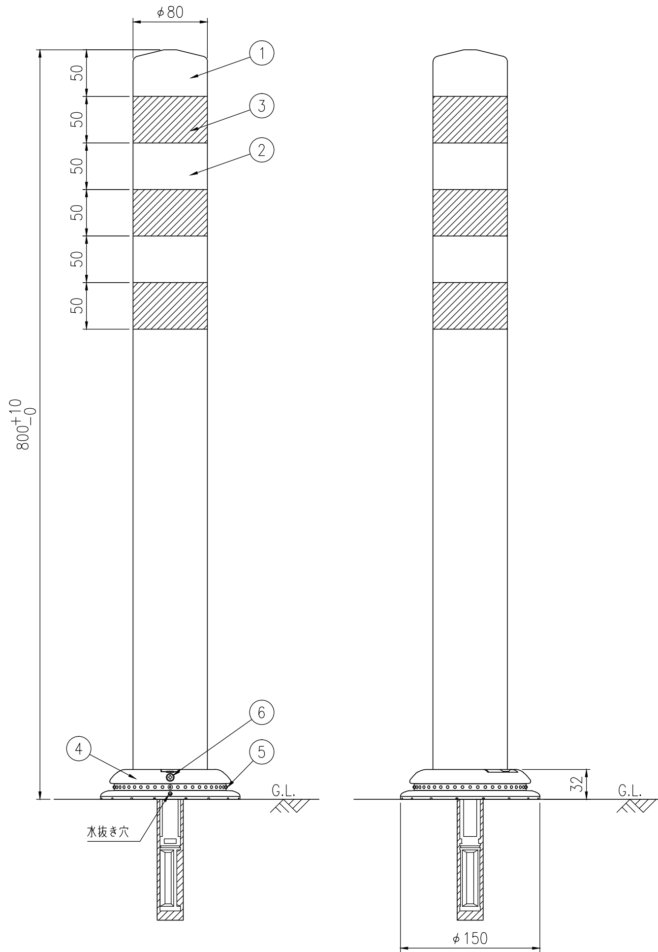
設置図 S=1/4
