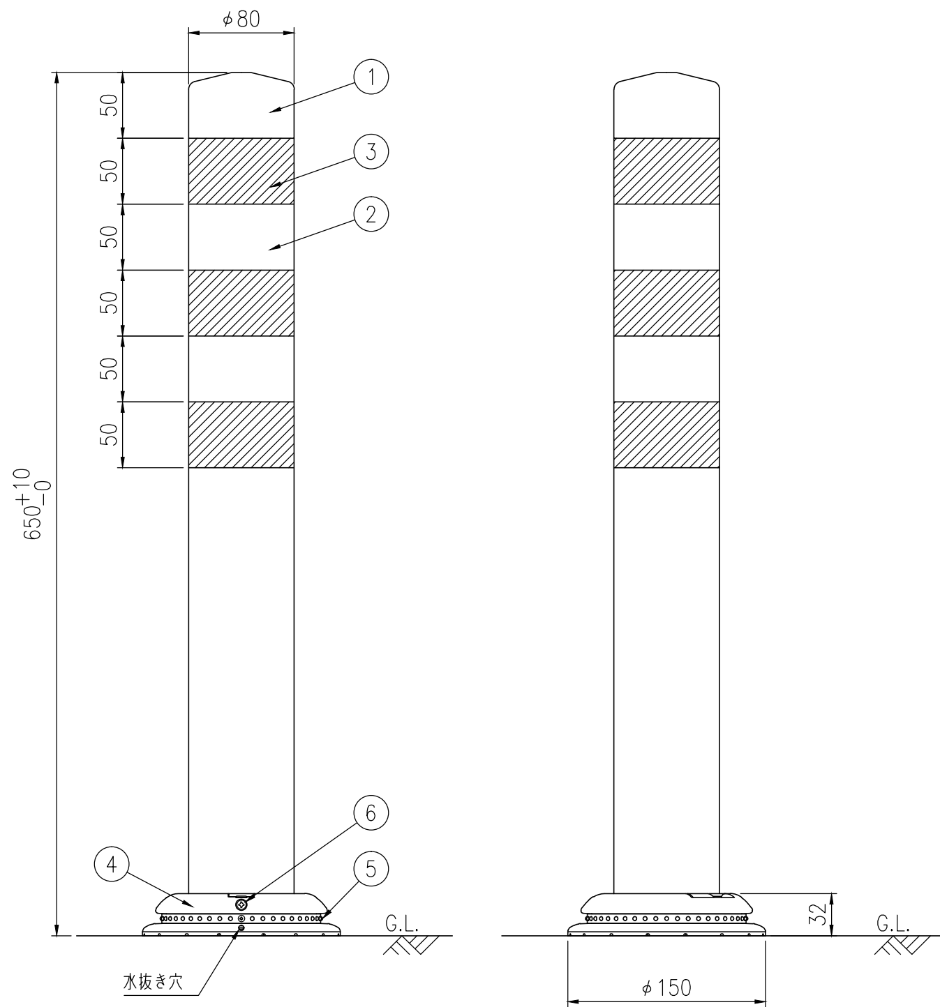
設置図 S=1/4
