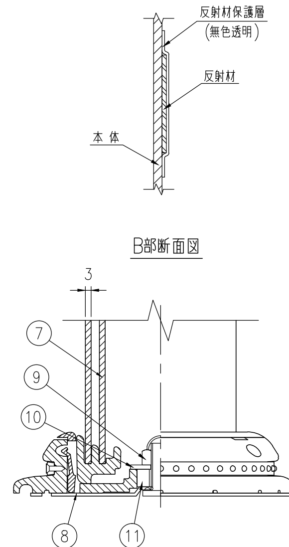
A-A半断面図 S=1/2
