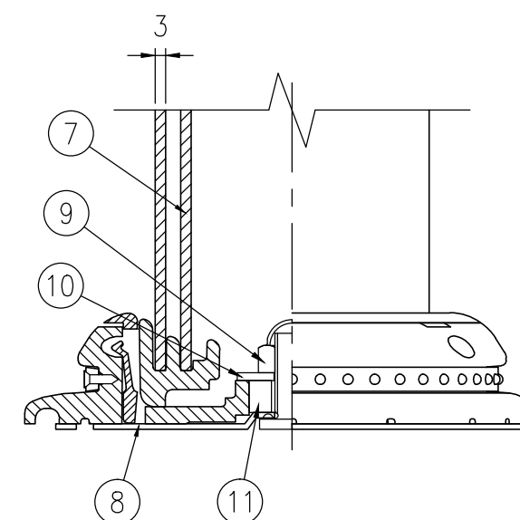
A-A半断面図 S=1/2
