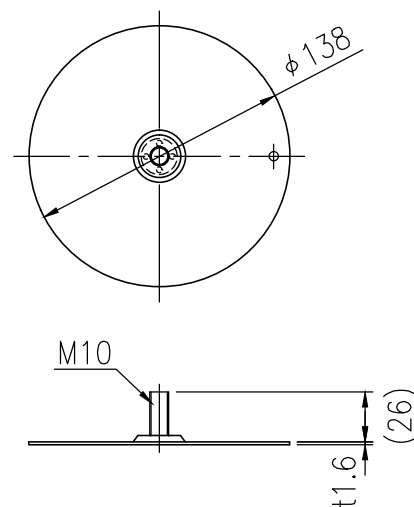
⑧ スチールスペーサー詳細図 S=1/4
