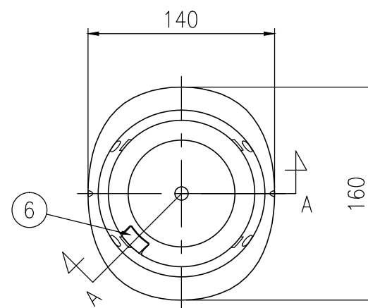
平面図 S=1/4
