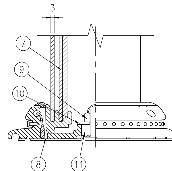
A-A半断面図 S=1/2
