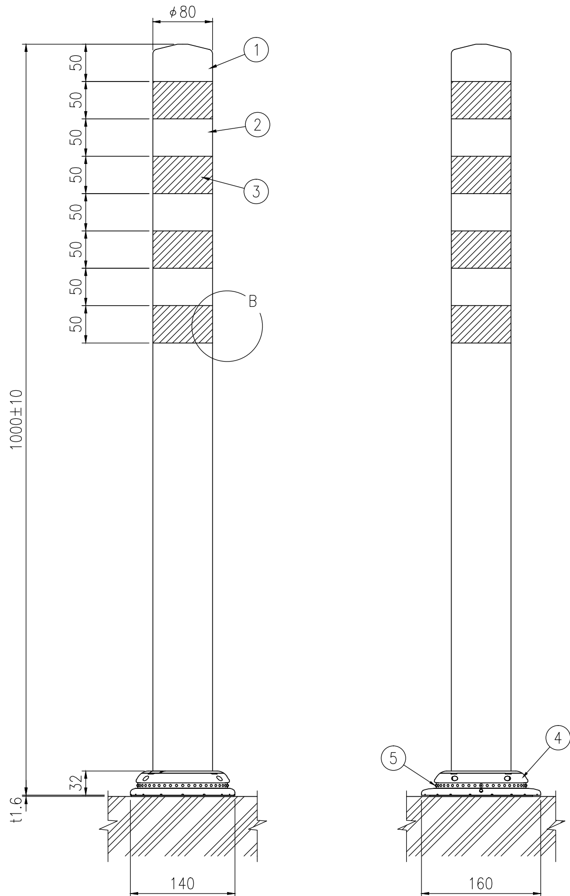
設置図 S=1/5
