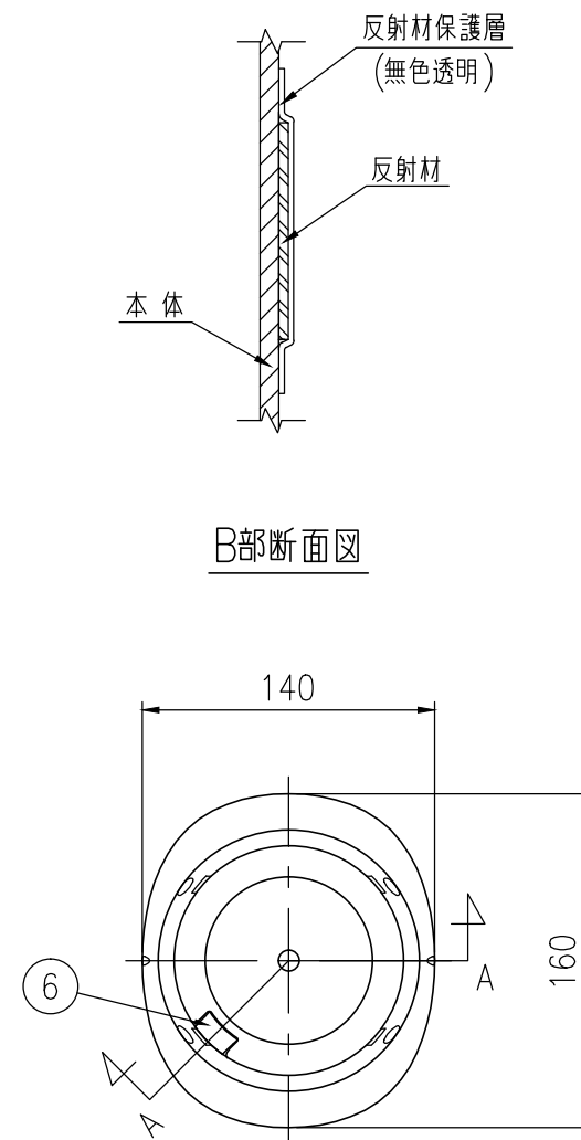
平面図 S=1/4
