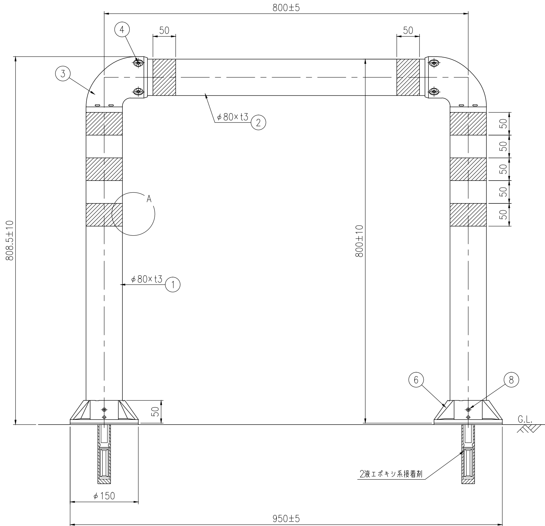
設置図 S=1/5
