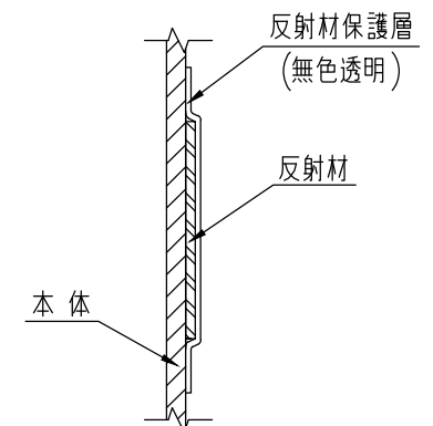
A部断面図
