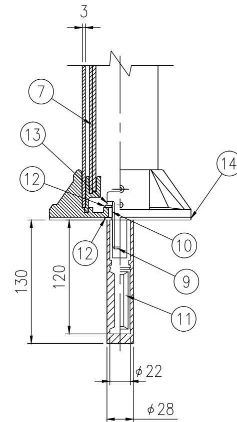
ベース部詳細図 S=1/4
