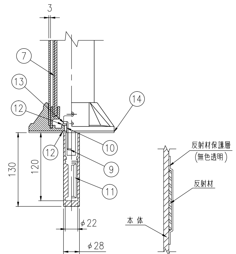
ベース部詳細図 S=1/4
