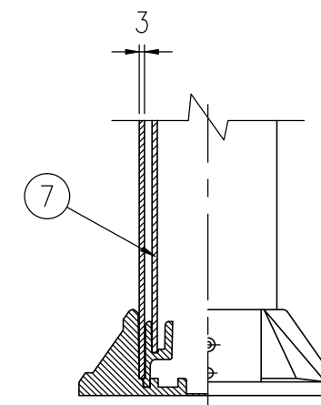
ベース部詳細図 S=1/4
