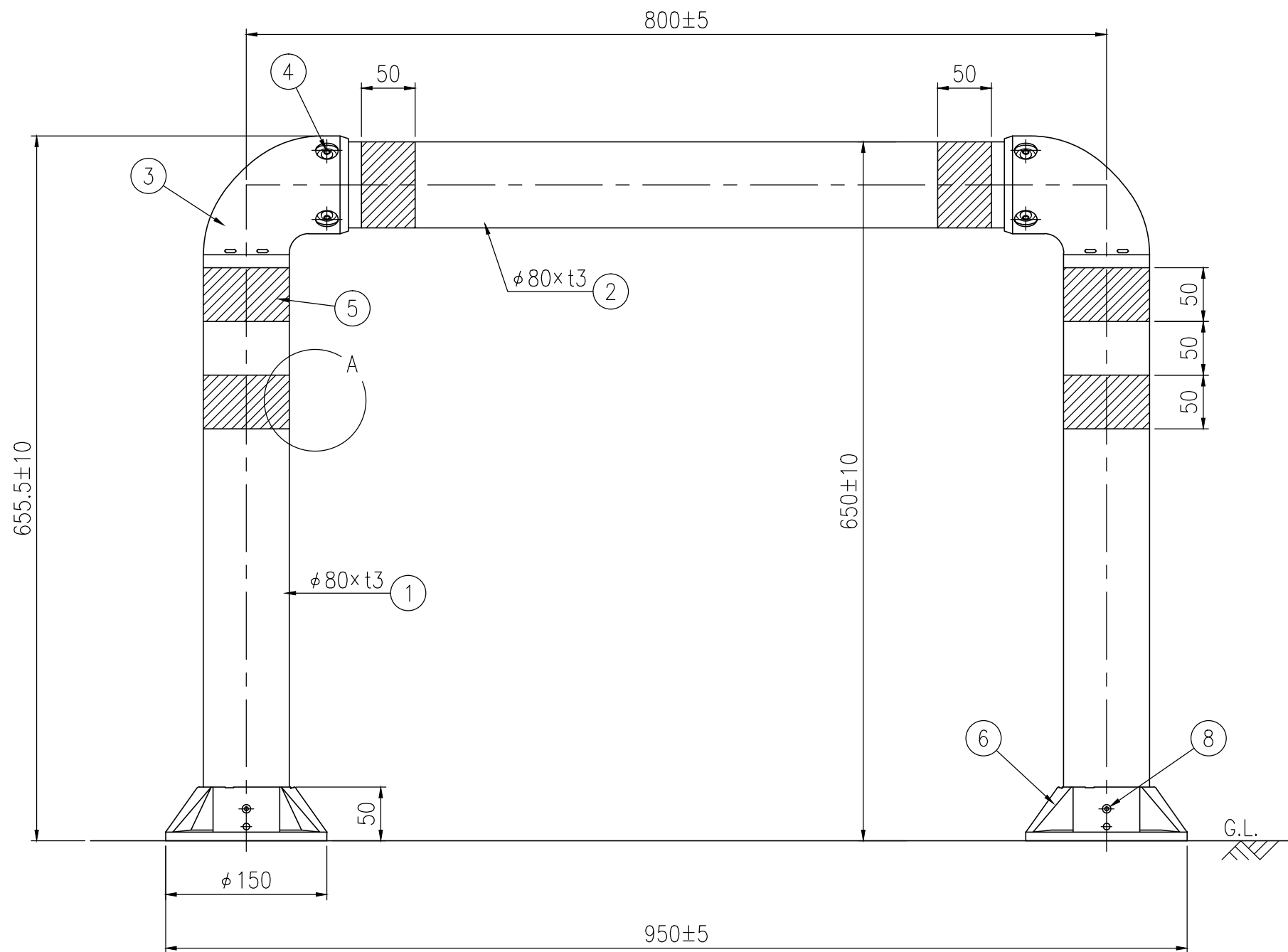
設置図 S=1/5
