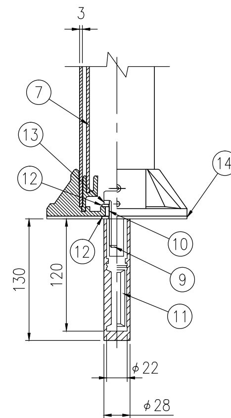
ベース部詳細図 S=1/4
