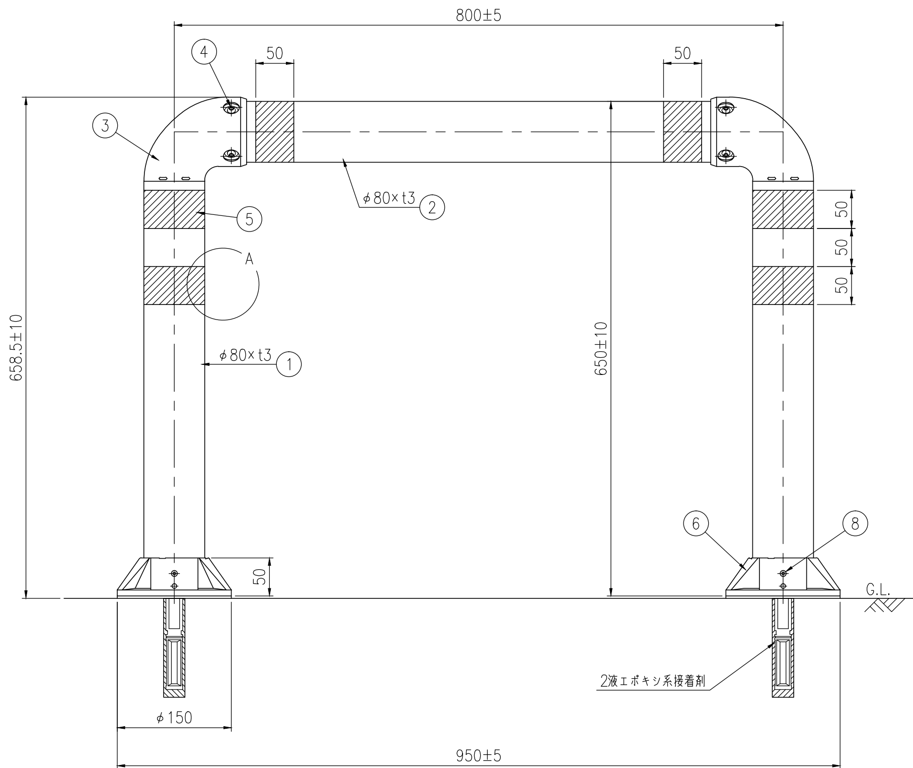
設置図 S=1/5
