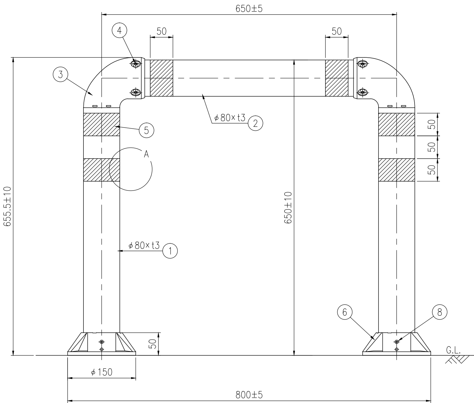
設置図 S=1/5
