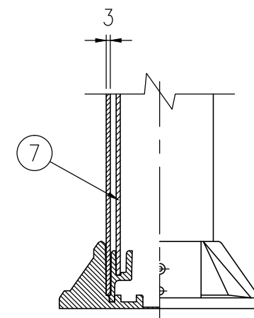
ベース部詳細図 S=1/4
