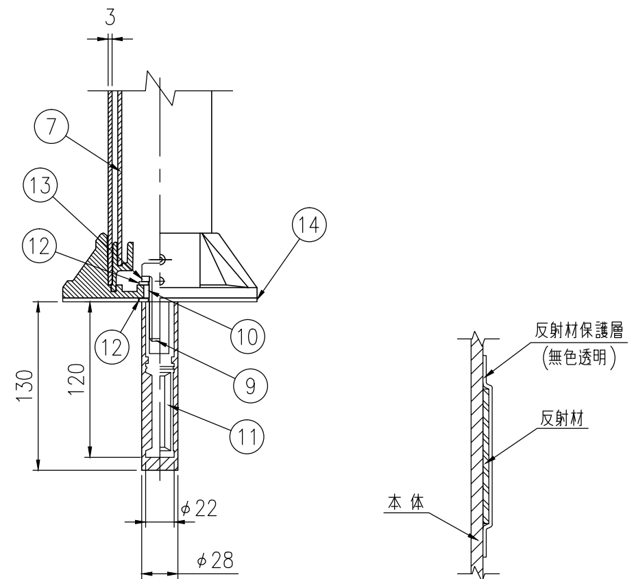
ベース部詳細図 S=1/4
