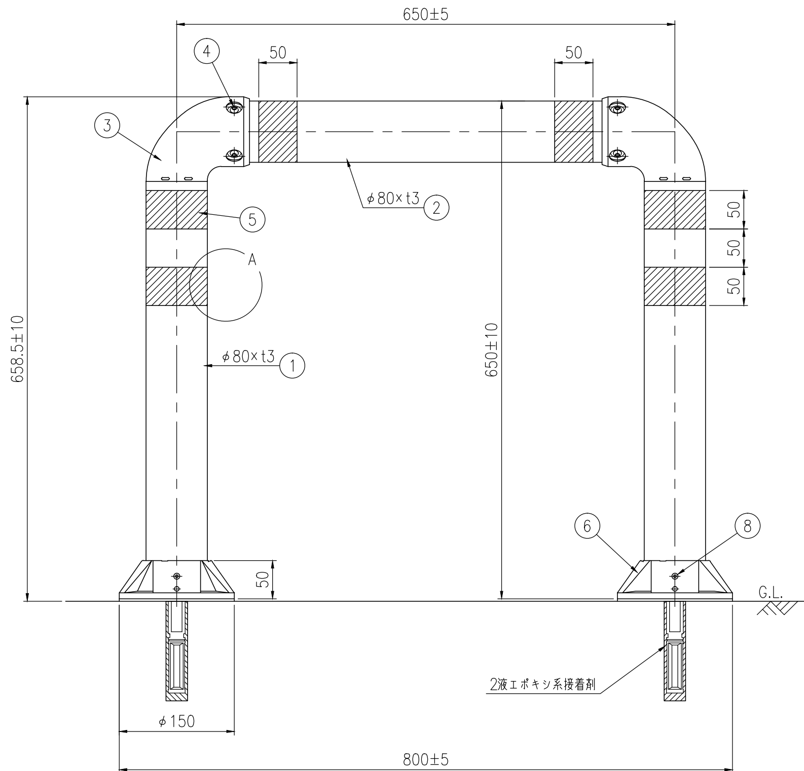
設置図 S=1/5
