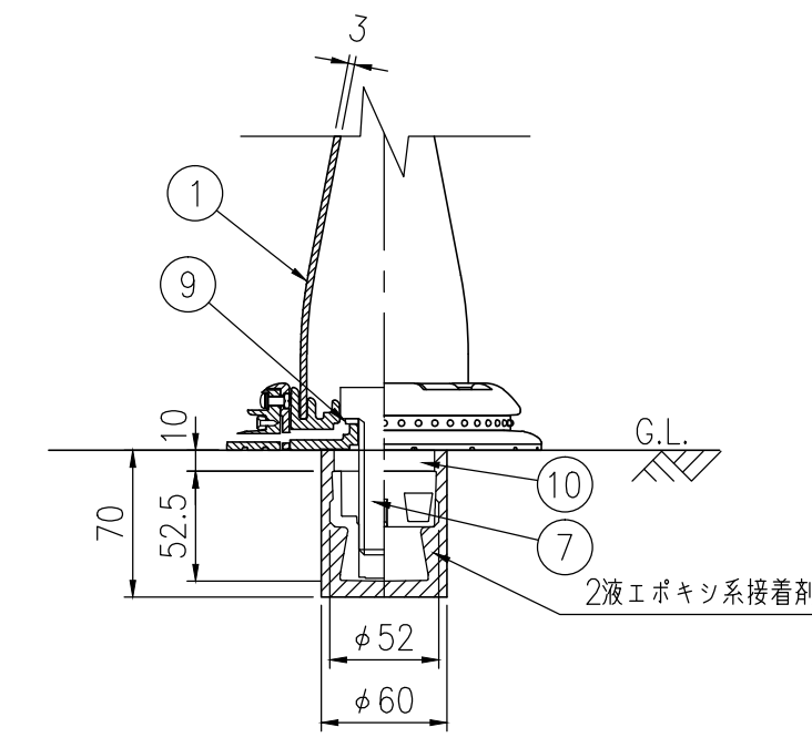
ベース部(設置図) S=1/4
