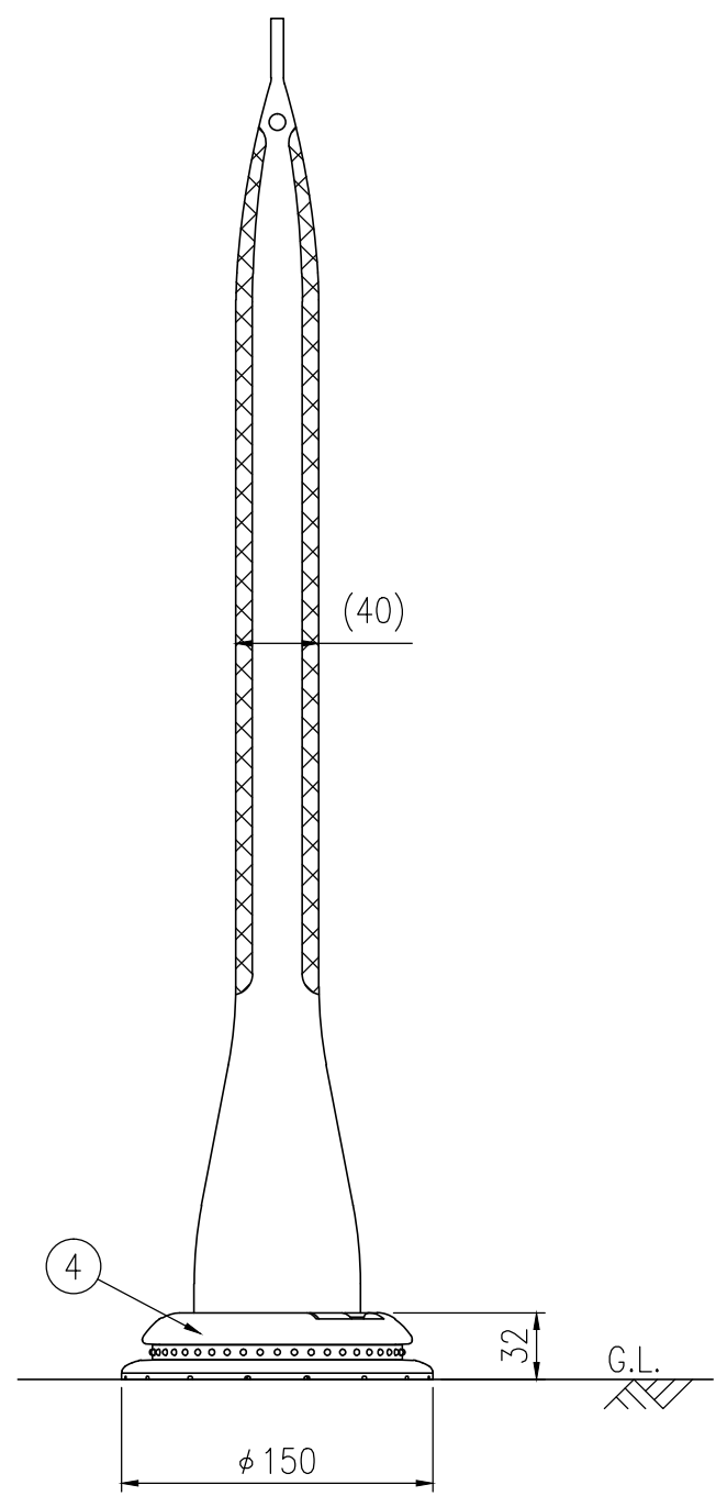
設置図 S=1/4
