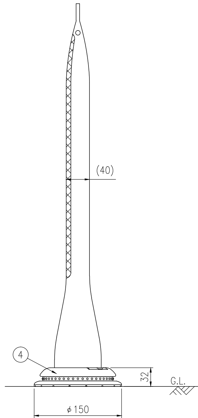
設置図 S=1/4
