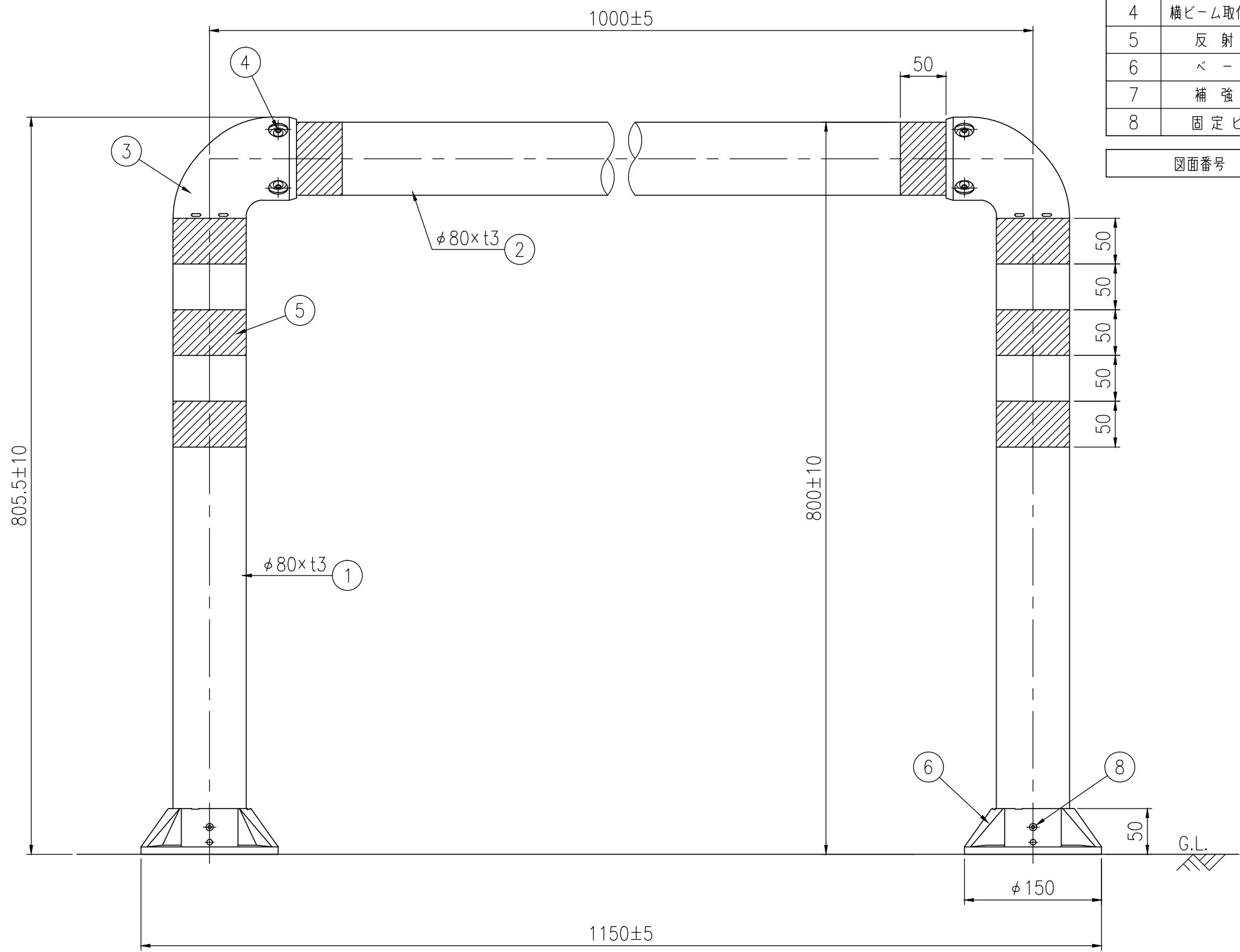
設置図 S=1/5
