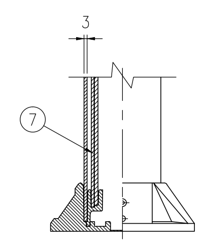
ベース部詳細図 S=1/4
