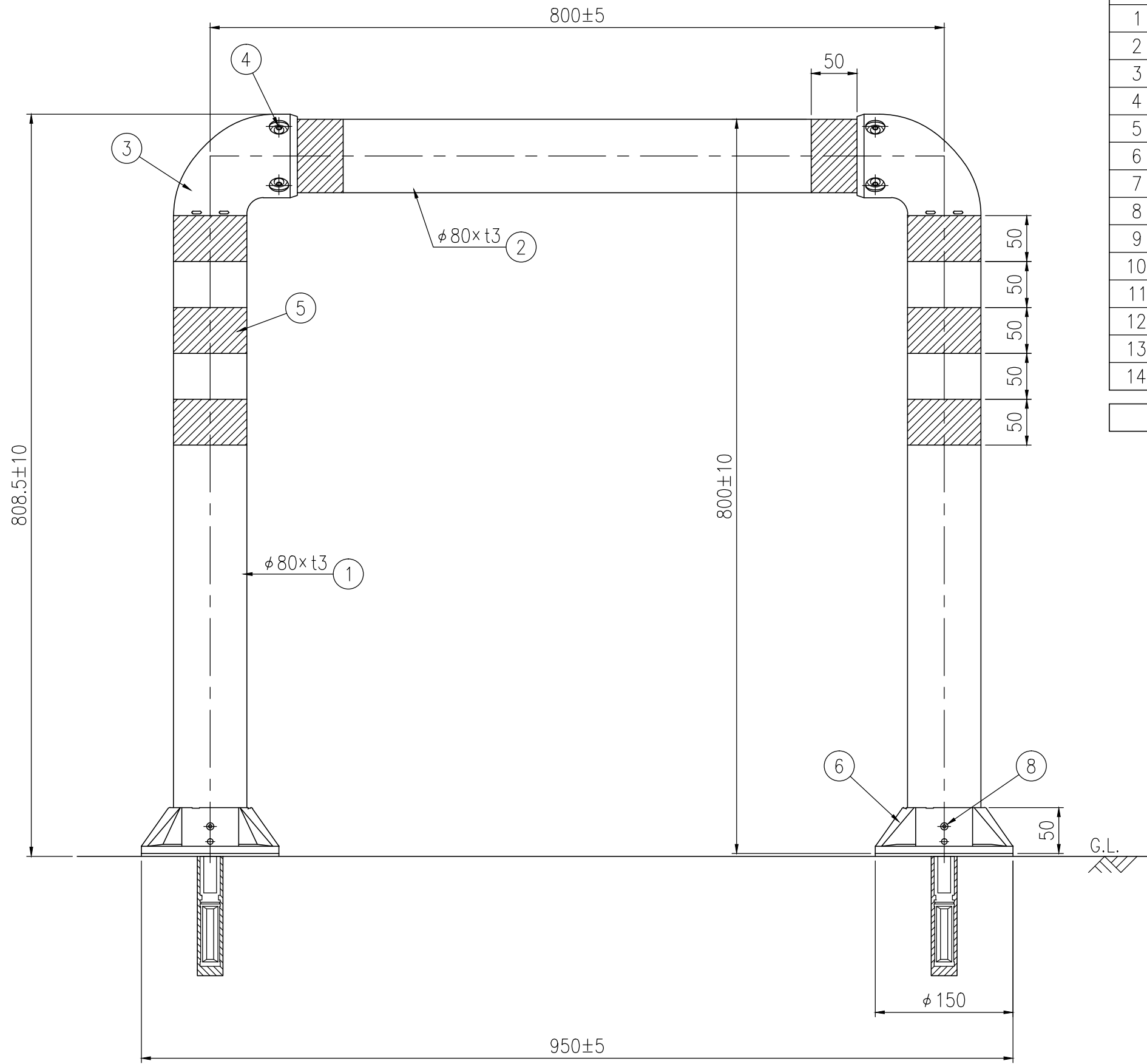
設置図 S=1/5
