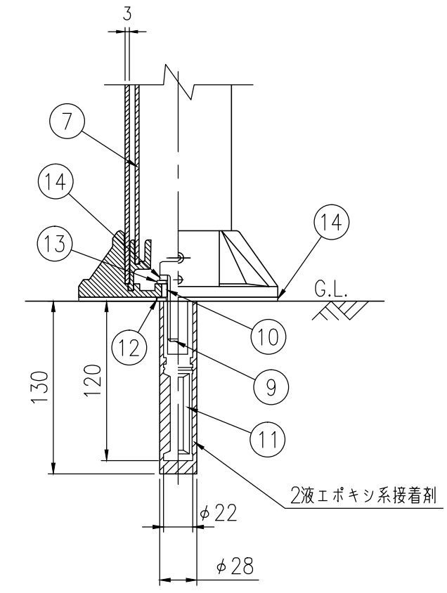
ベース部詳細図 S=1/4
