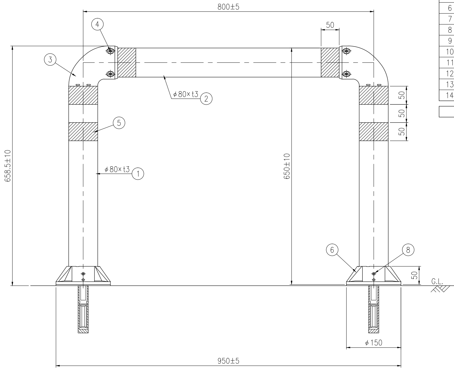
設置図 S=1/5
