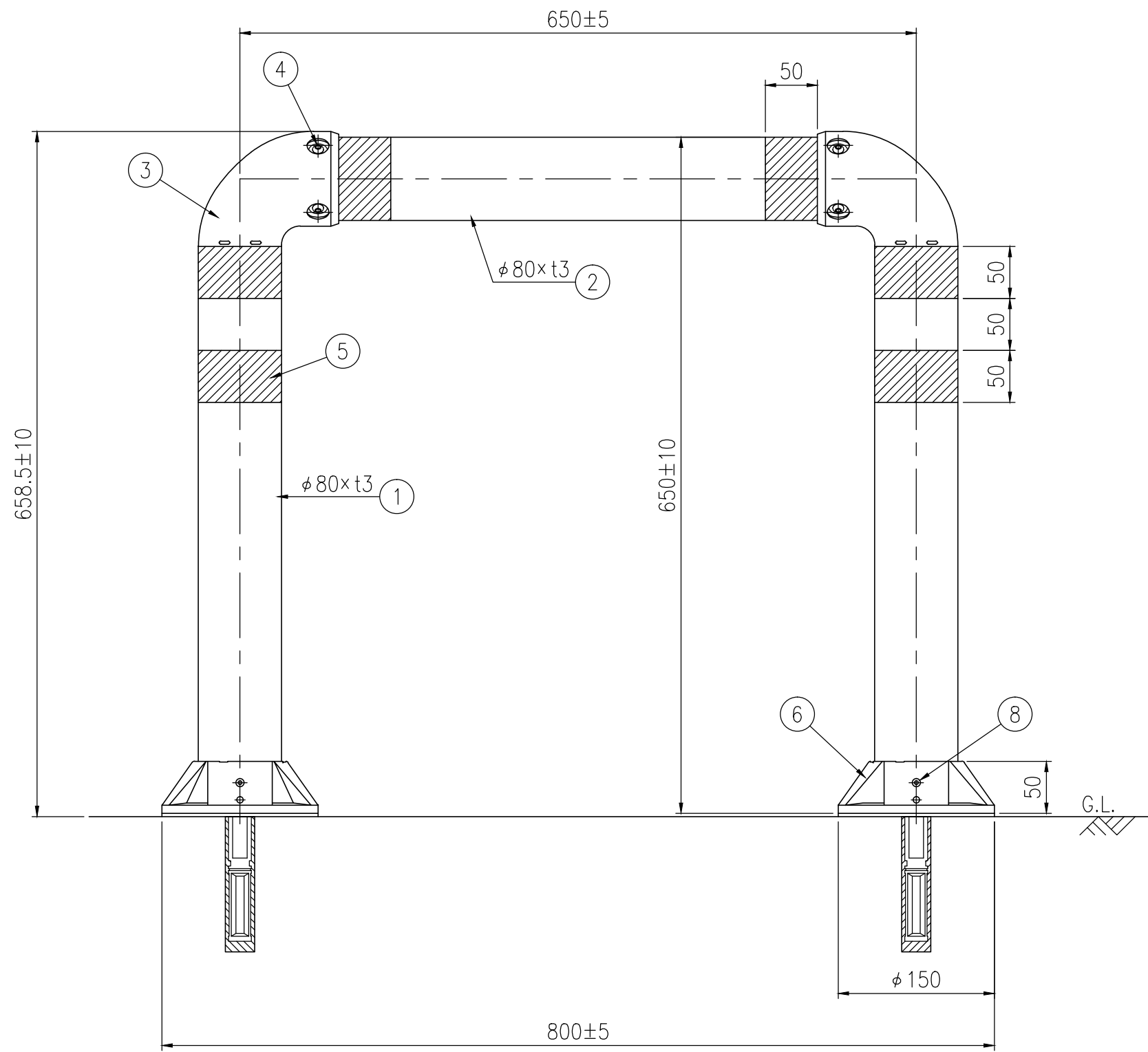
設置図 S=1/5
