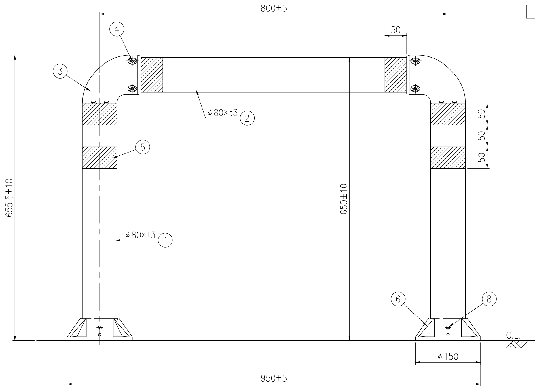
設置図 S=1/5
