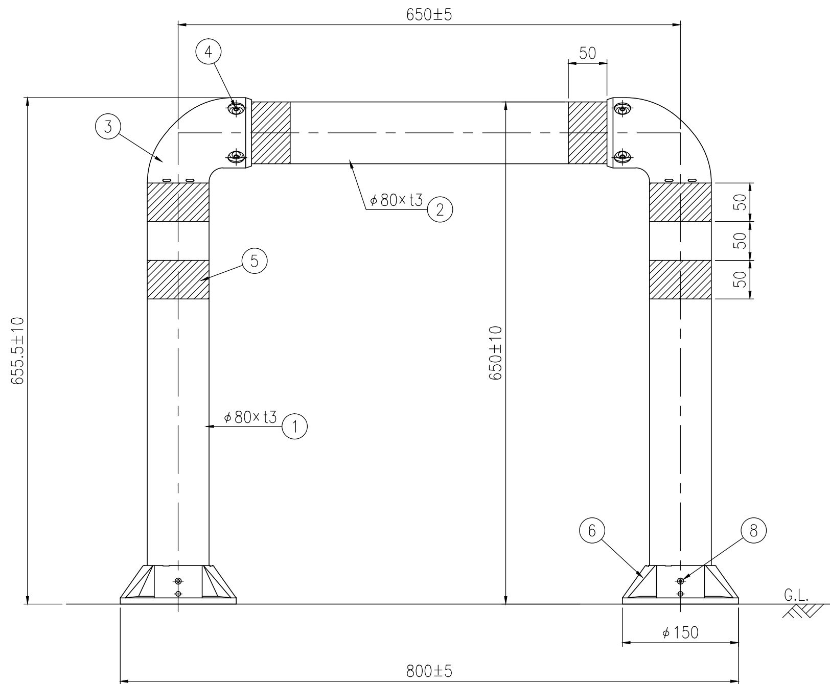
設置図 S=1/5
