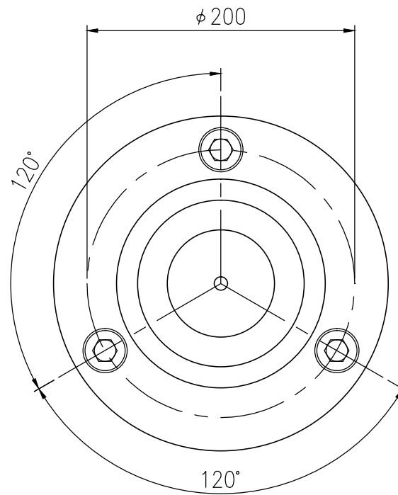
上面図 S=1/4
