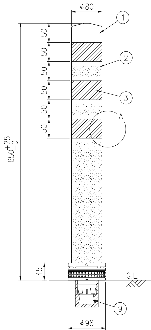
設置図 S=1/5
