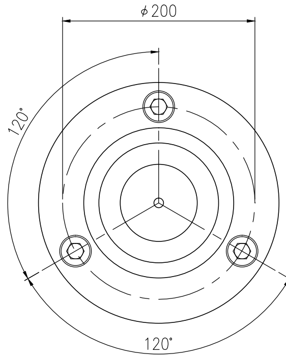
上面図 S=1/4
