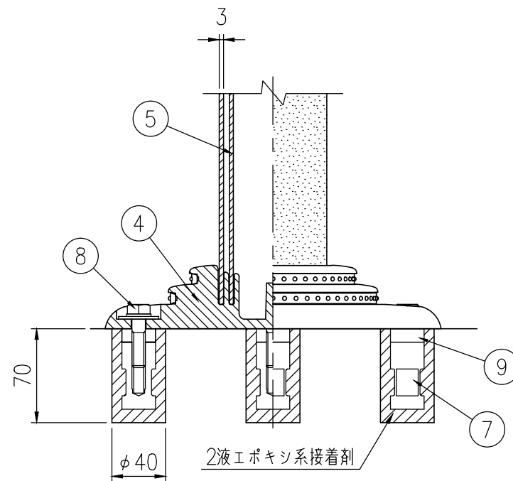
ベース部詳細図 S=1/4
