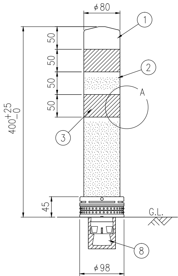
設置図 S=1/5
