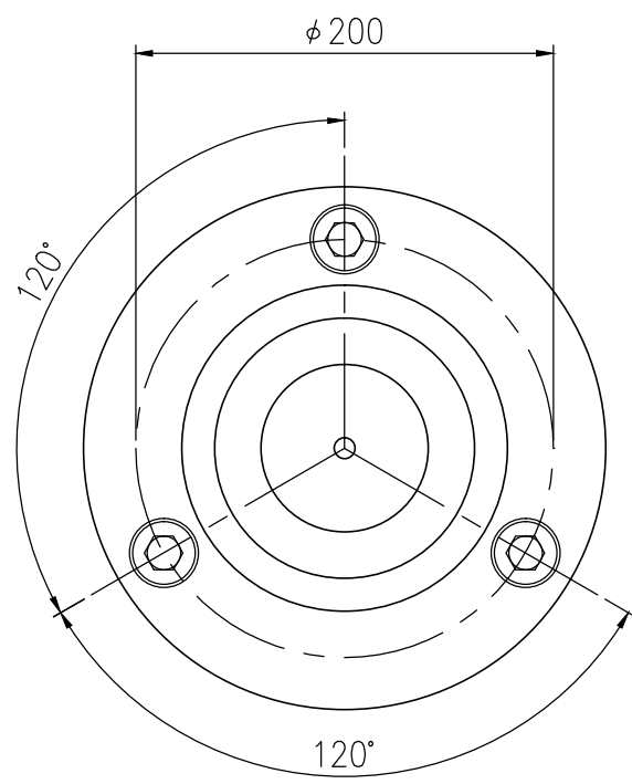
上面図 S=1/4
