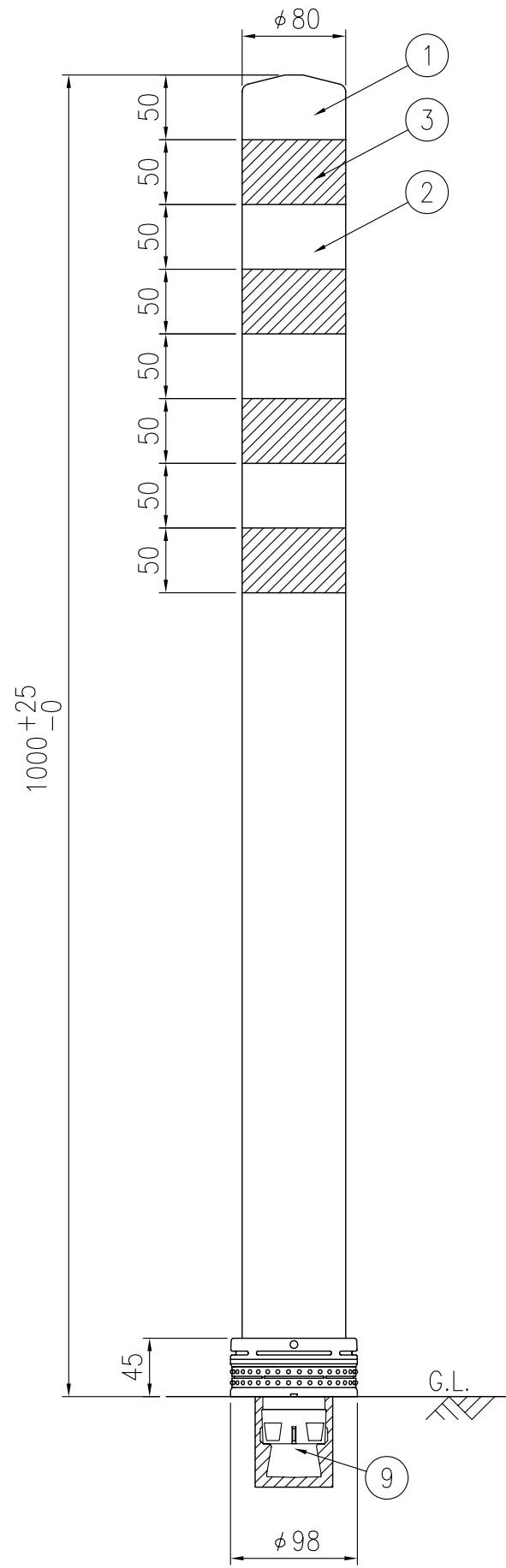
設置図 S=1/5
