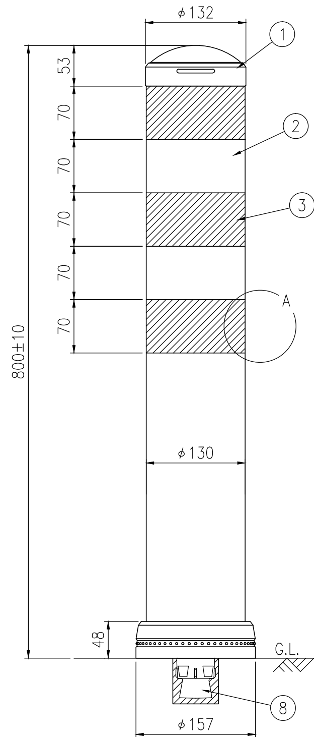
設置図 S=1/5
