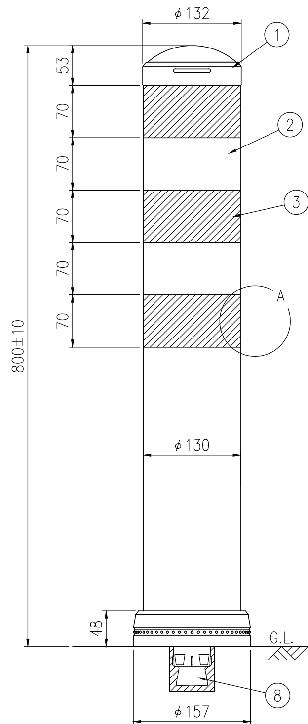
設置図 S=1/5
