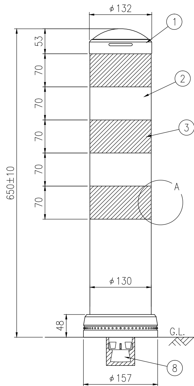
設置図 S=1/5
