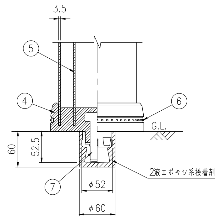
ベース部詳細図 S=1/4
