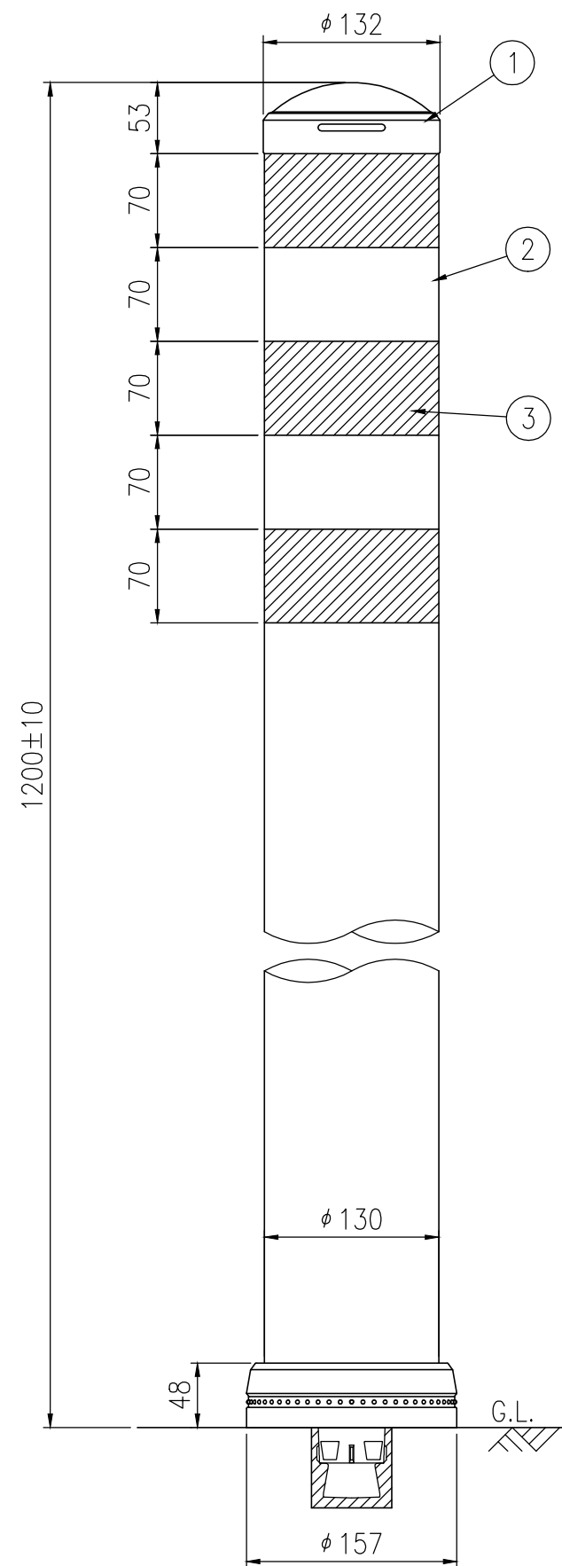
設置図 S=1/5
