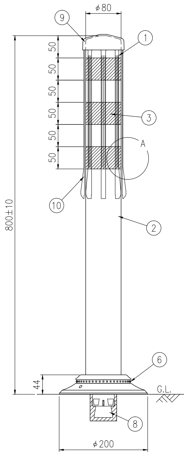
設置図 S=1/5
