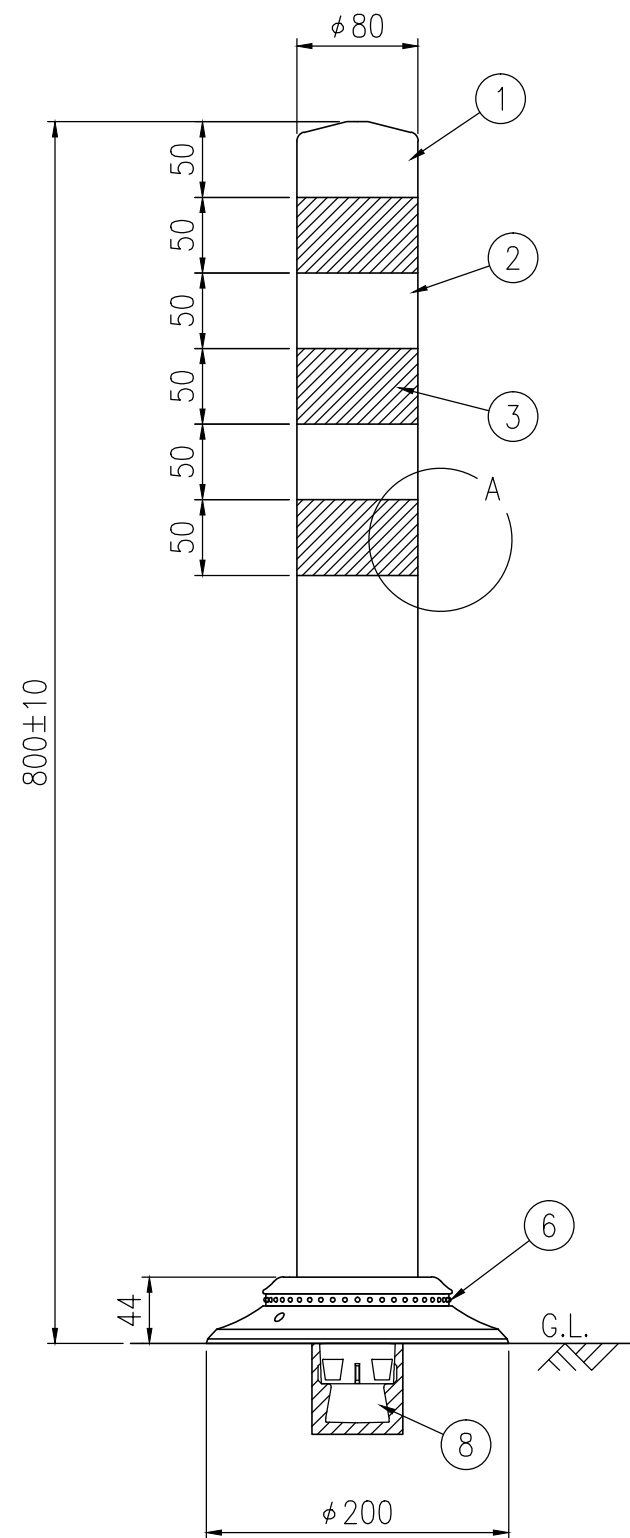
設置図 S=1/5
