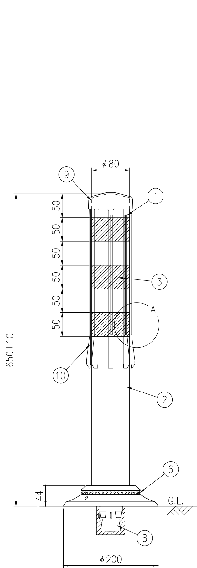
設置図 S=1/5
