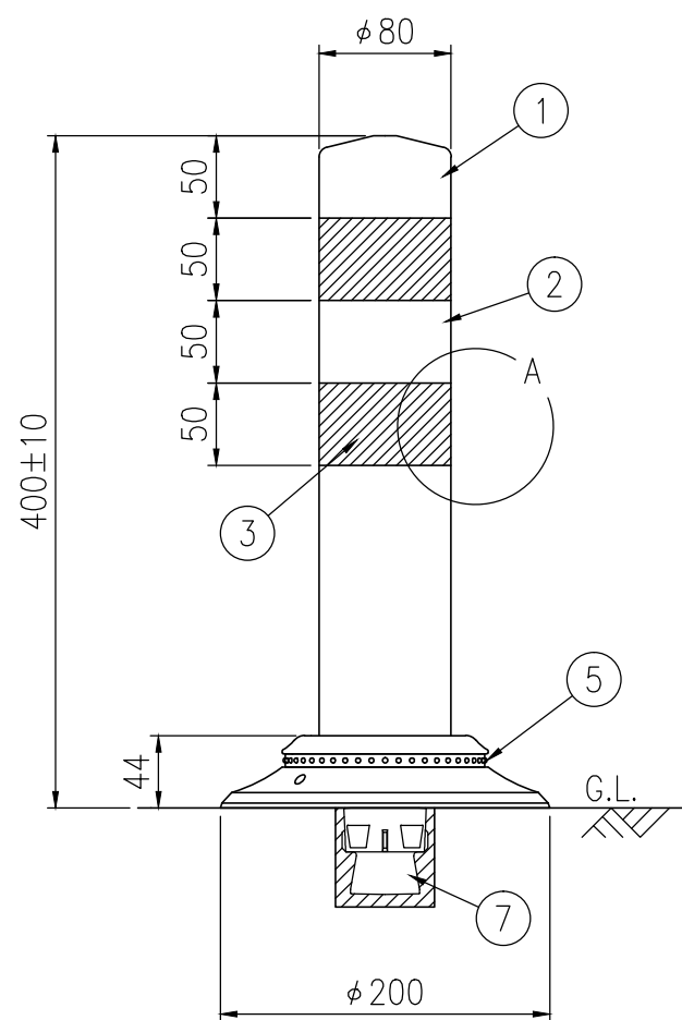
設置図 S=1/5
