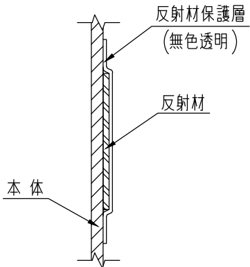
A部断面図
