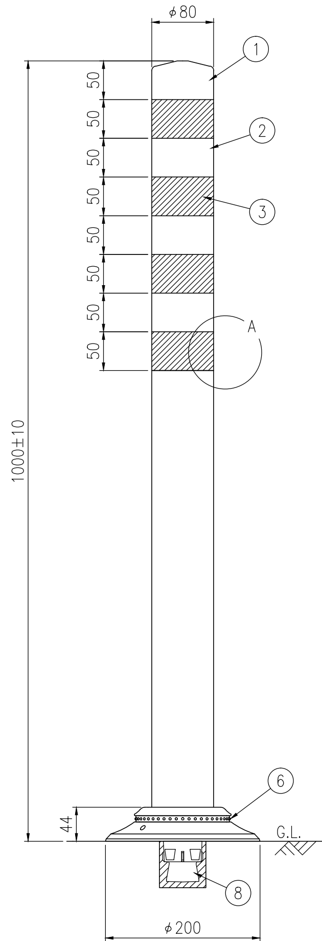
設置図 S=1/5
