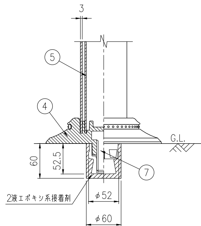
ベース部詳細図 S=1/4
