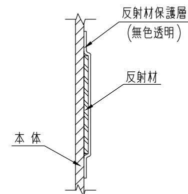
A部断面図
