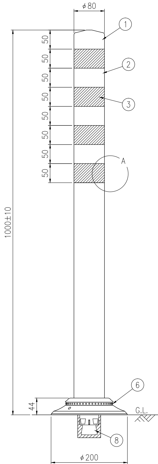
設置図 S=1/5
