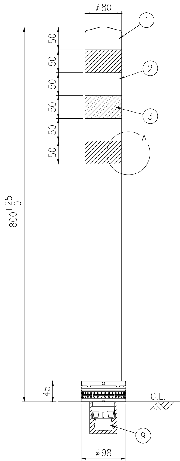
設置図 S=1/5
