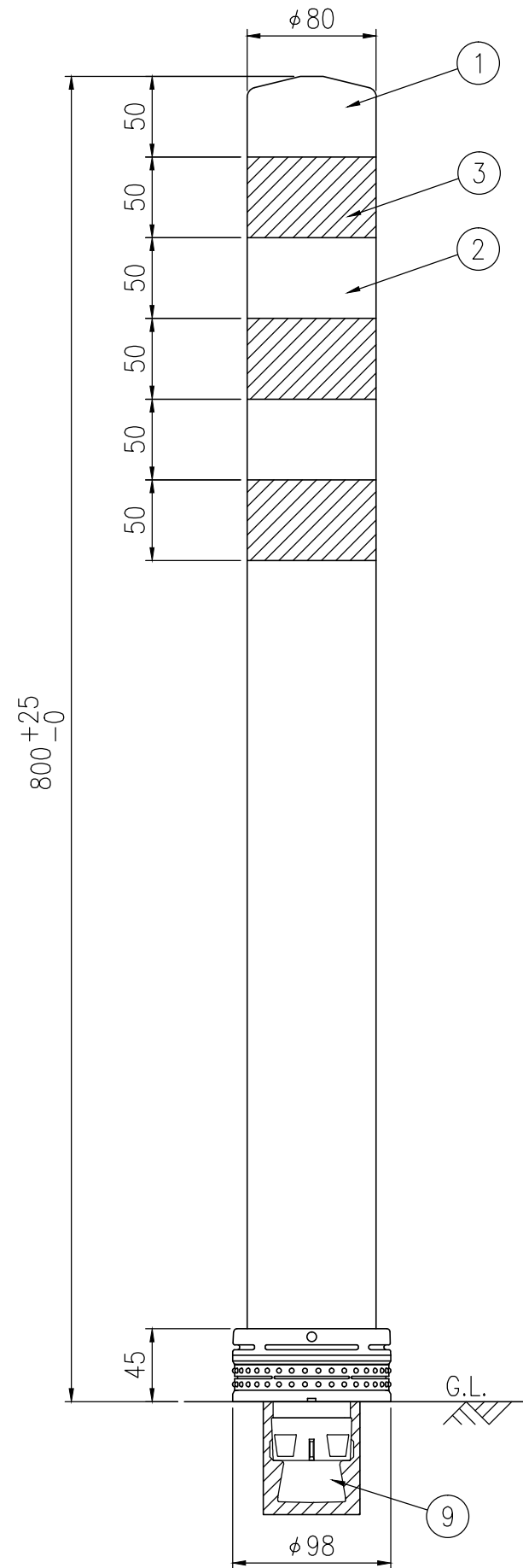
設置図 S=1/4
