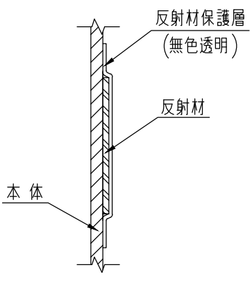
A部断面図
