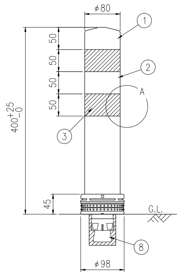
設置図 S=1/5
